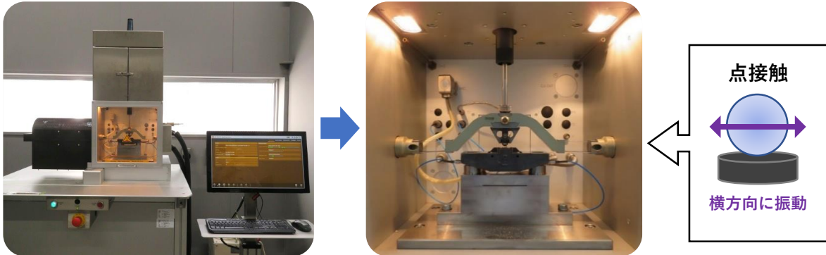
◆SRV試験機
