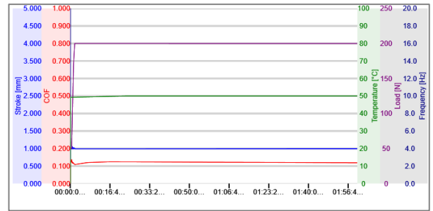
◆摩耗特性(Wear)データ（例）
